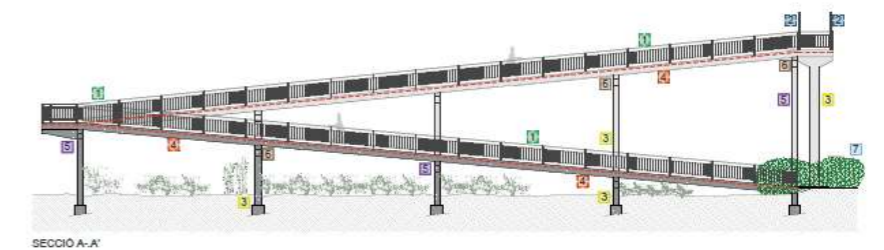
SECCIÓ A-A'
